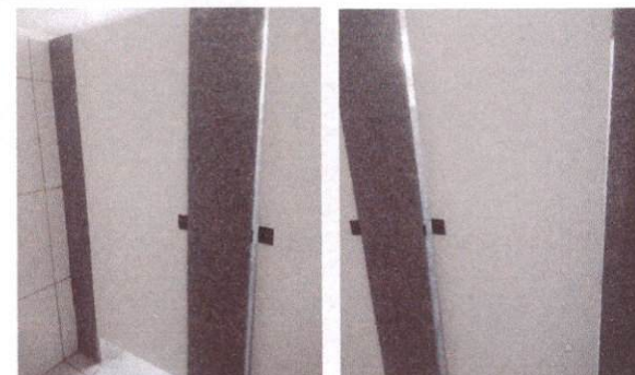
6.1.3/6.2.3 PM3 - Porta em compensado de madeira, dimensões 90x160cm, folha lisa revestida com laminado melamínico; incluso marco e dobradiças/Fechadura de embutir completa, tipo tarjeta livre-ocupado
