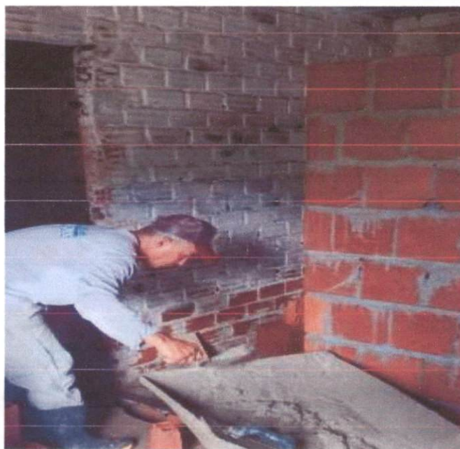
Item: 5.2; ALVENARIA EM PEDRA RACHAO ASSENTADA E REJUNTA DA COM ARGAMASSA DE CIMENTO E AREIA NO TRACO 1:6. BASE DA RAMPA
